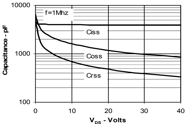
Fig. 11. Capacitance
